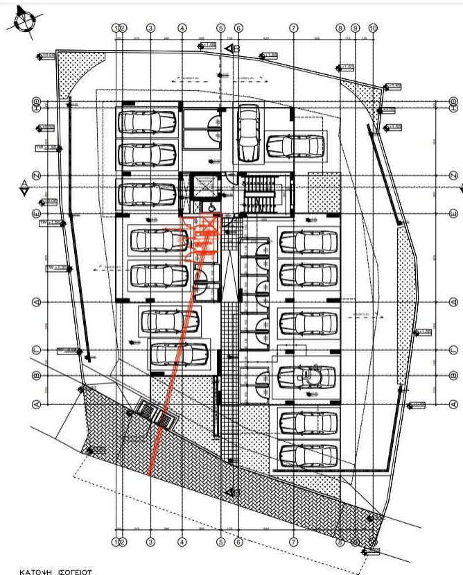
ΚΑΤΩΗ ΙΣΟΓΕΙΟΥ
