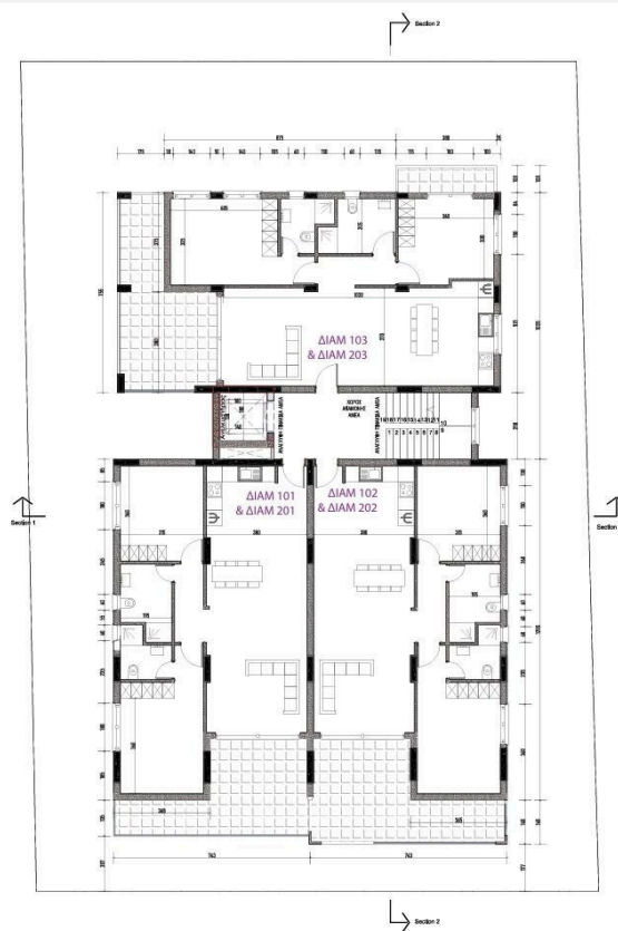
ΚΑΤΟΨΗ 1ου και 2ου ΟΡΟΦΟΥ
