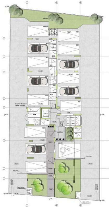
ΚΑΤΟΨΗ ΙΣΟΓΕΙΟΥ
