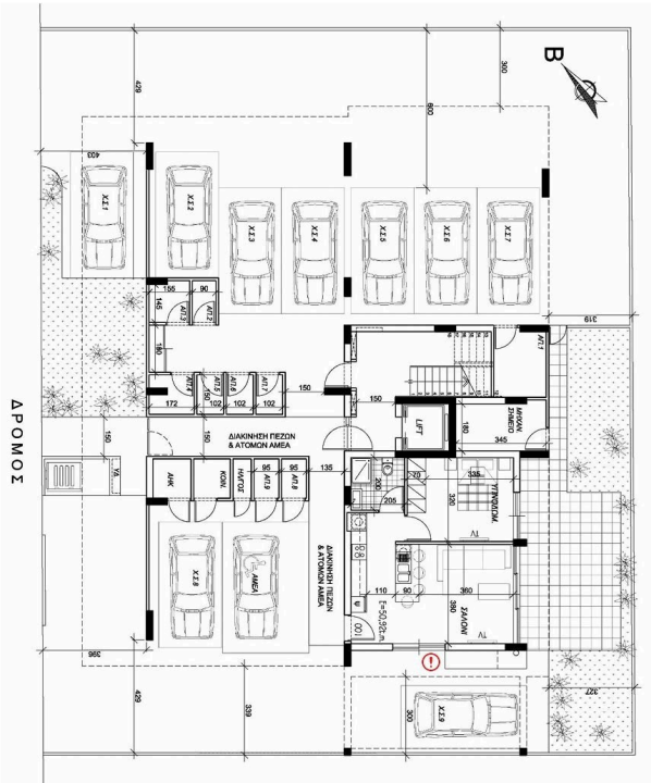
ΙΣΟΓΕΙΟ - ΠΥΛΩΤΗ
