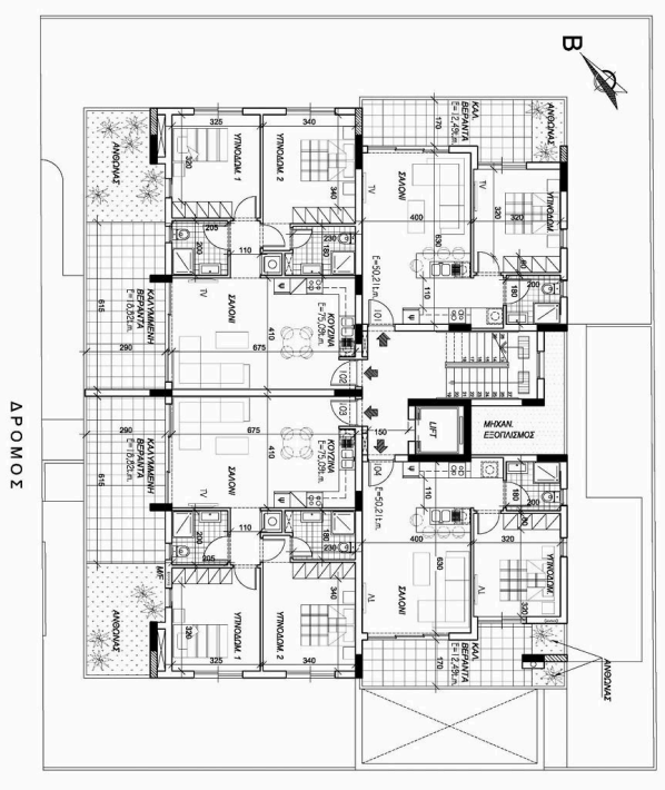
1 ος ΟΡΟΦΟΣ
