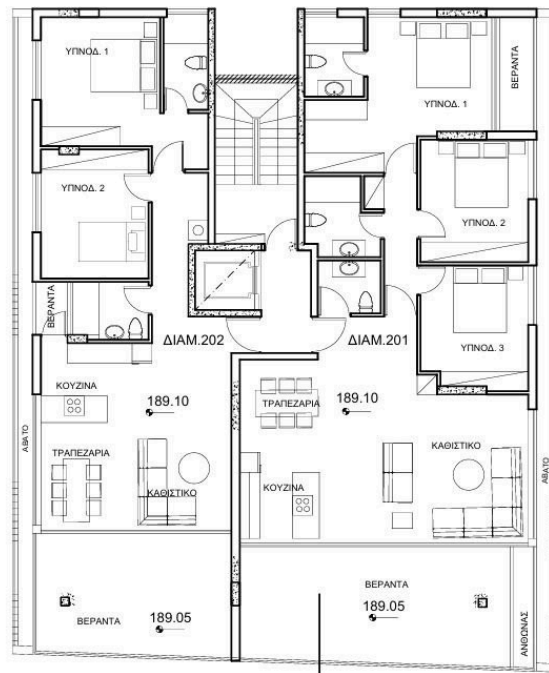
ΚΑΤΟΨΗ 2ου ΟΡΟΦΟΥ
