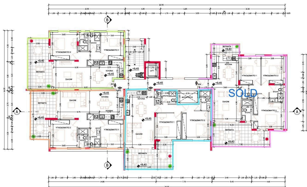
ΚΑΤΩΦΗ 3ου ΟΡΟΦΟΥ ΚΛΙΜΑΚΑ 1:100
