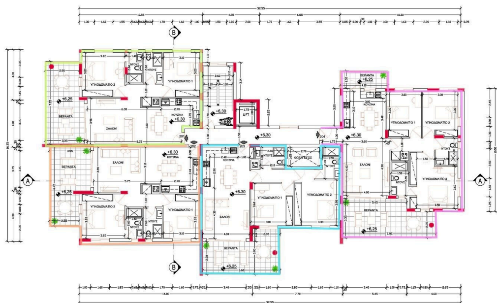
ΚΑΤΩΦΗ 2ου ΟΡΟΦΟΥ ΚΛΙΜΑΚΑ 1:100
