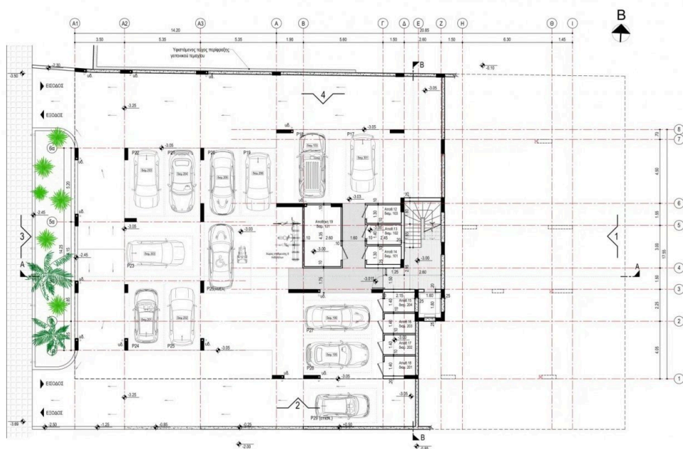
ΚΑΤΩΦΗ ΥΠΟΓΕΙΟΥ
