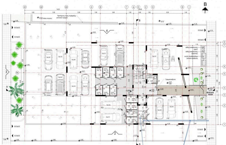
ΚΑΤΩΦΗ ΙΣΟΓΕΙΟΥ
