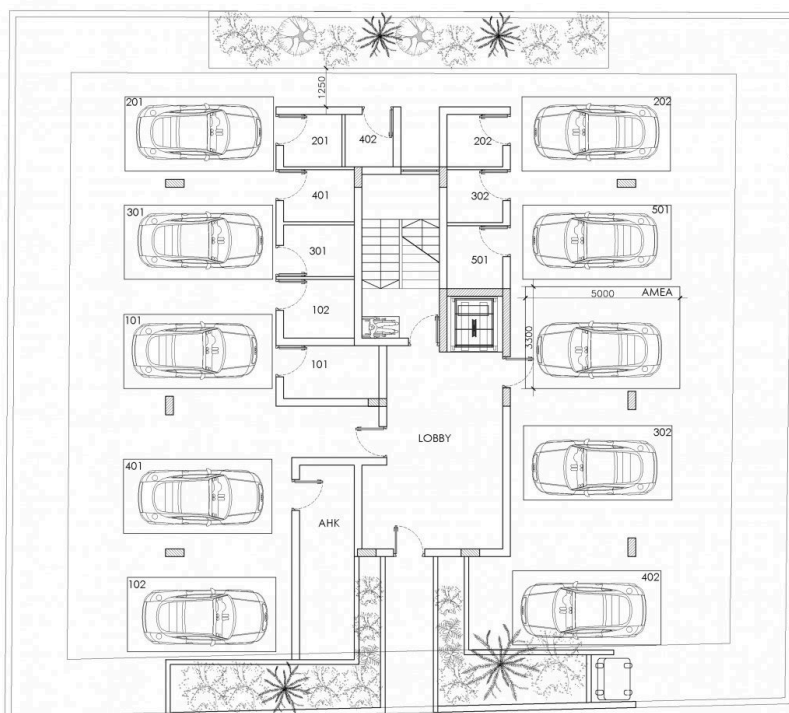
ΚΑΤΟΨΗ ΙΣΟΓΕΙΟΥ 1:100@A3
