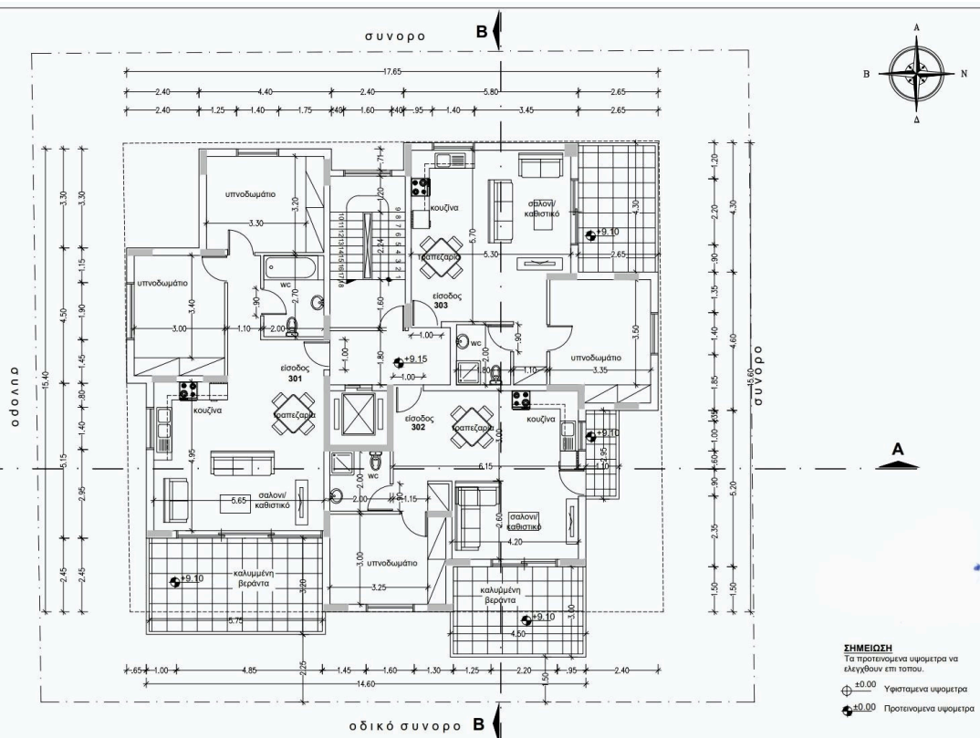
ΚΑΤΩΨΗ 3ου ΟΡΟΦΟΥ ΚΛΙΜΑΚΑ 1:100
