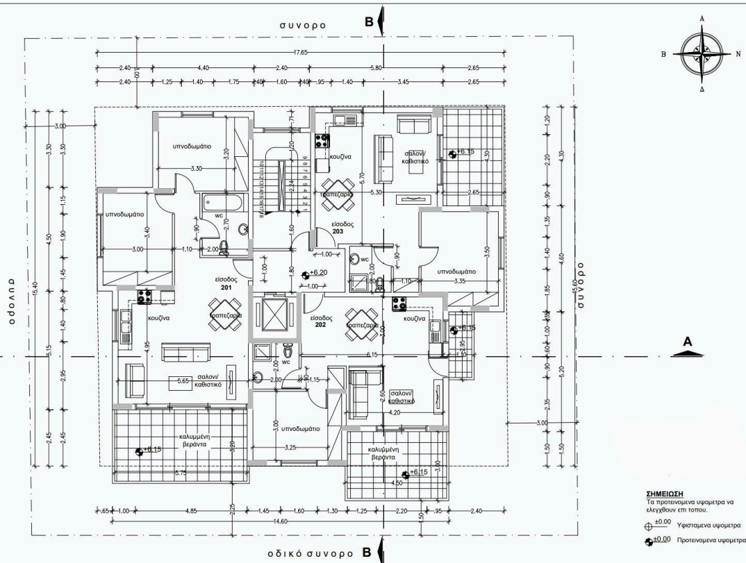
ΚΑΤΩΨΗ 2ου ΟΡΟΦΟΥ ΚΛΙΜΑΚΑ 1:100
