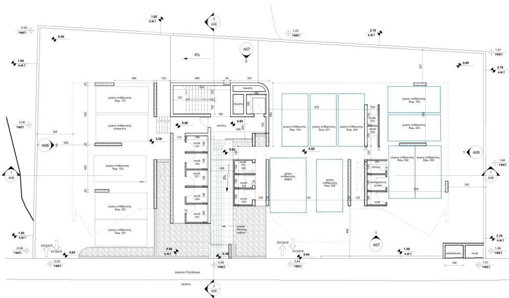
01-Κάτοψη Ισογείου 1 : 100
