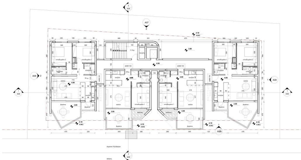
02-Κάτοψη 1ου Ορόφου 1 : 100
