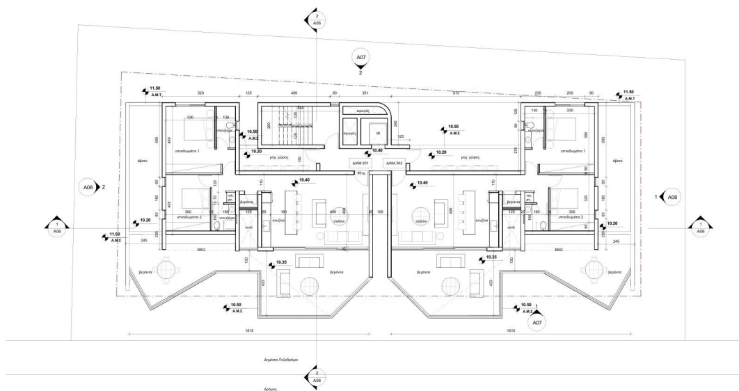
04-Κάτοψη 3ου Ορόφου 1: 100
