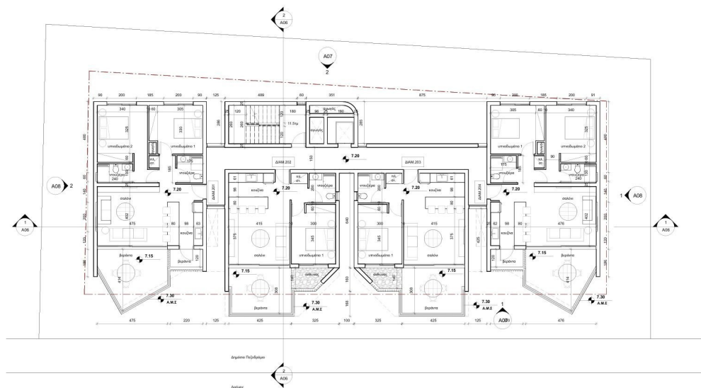
03-Κάτοψη 2ου Ορόφου 1: 100
