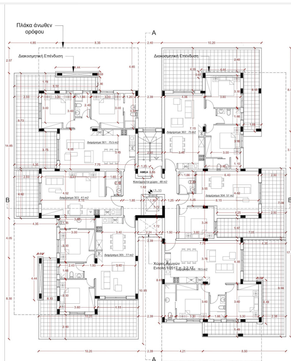
Κάτοψη 3ου Ορόφου
