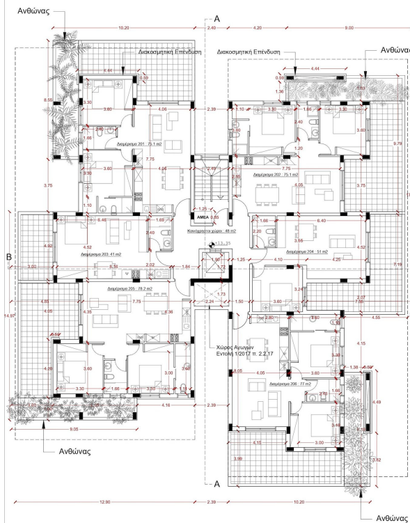
Κάτοψη 4ου Ορόφου
