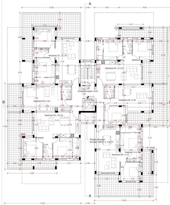
Κάτοψη 2ου Ορόφου
