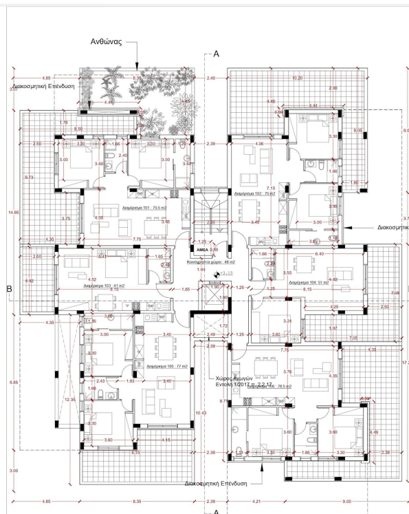
Κάτοψη 1ου Ορόφου
