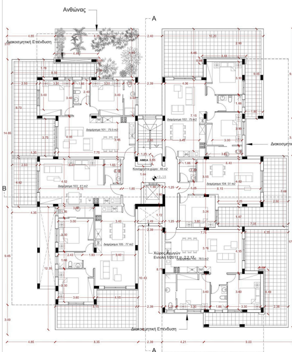
Κάτοψη 1ου Ορόφου
