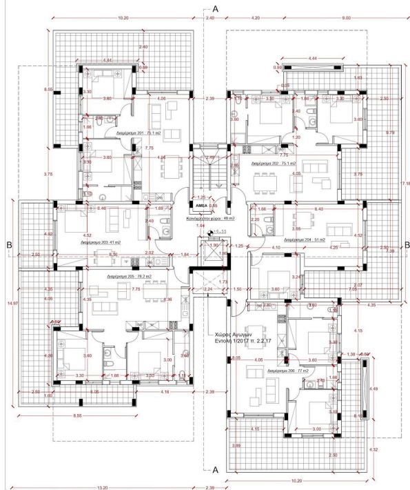
Κάτοψη 2ου Ορόφου
