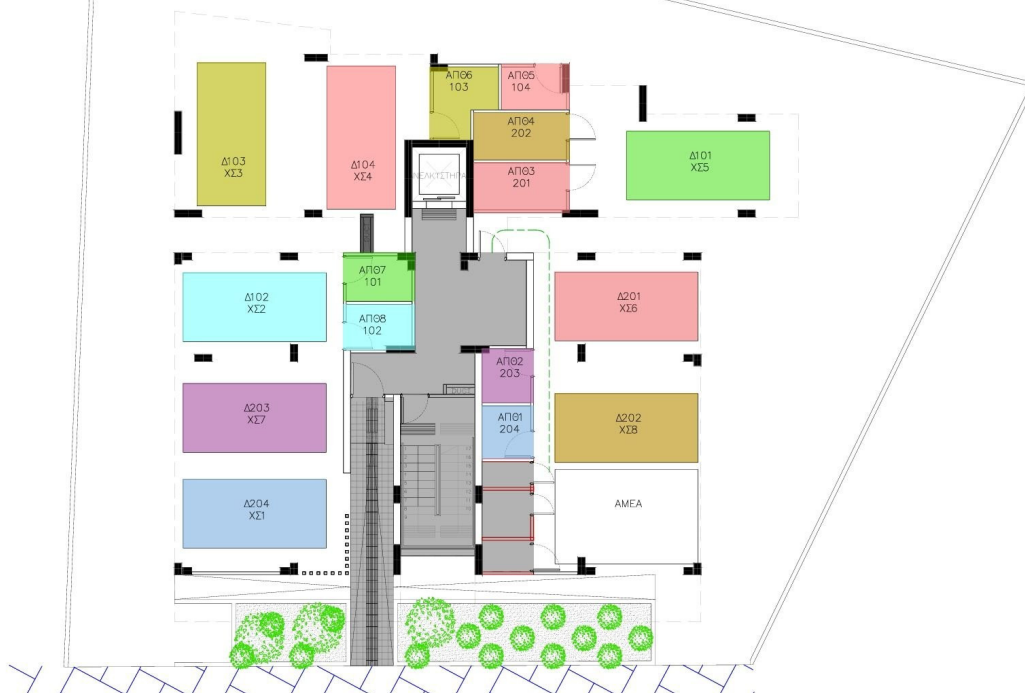
ΚΑΤΟΨΗ ΙΣΟΓΕΙΟΥ
