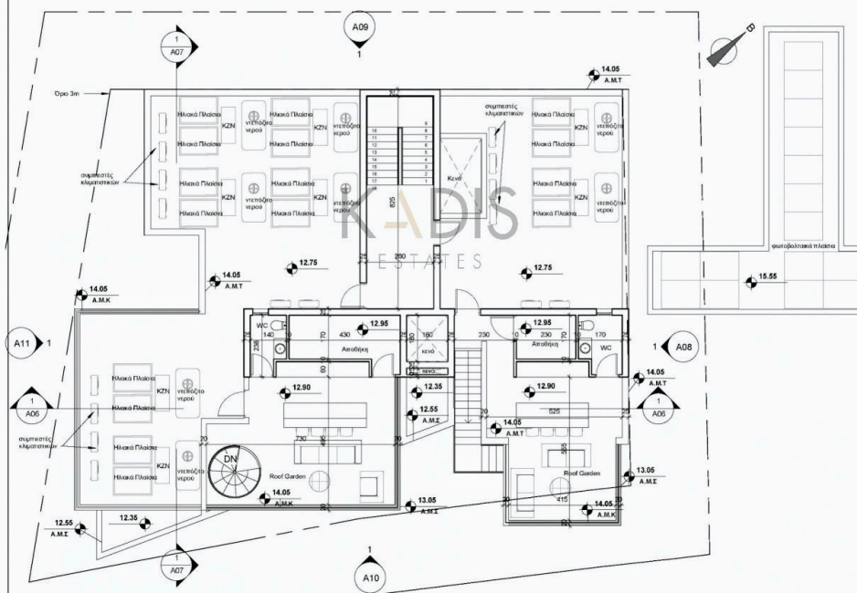
1 04-Κάτοψη Οροφής 1 : 100
