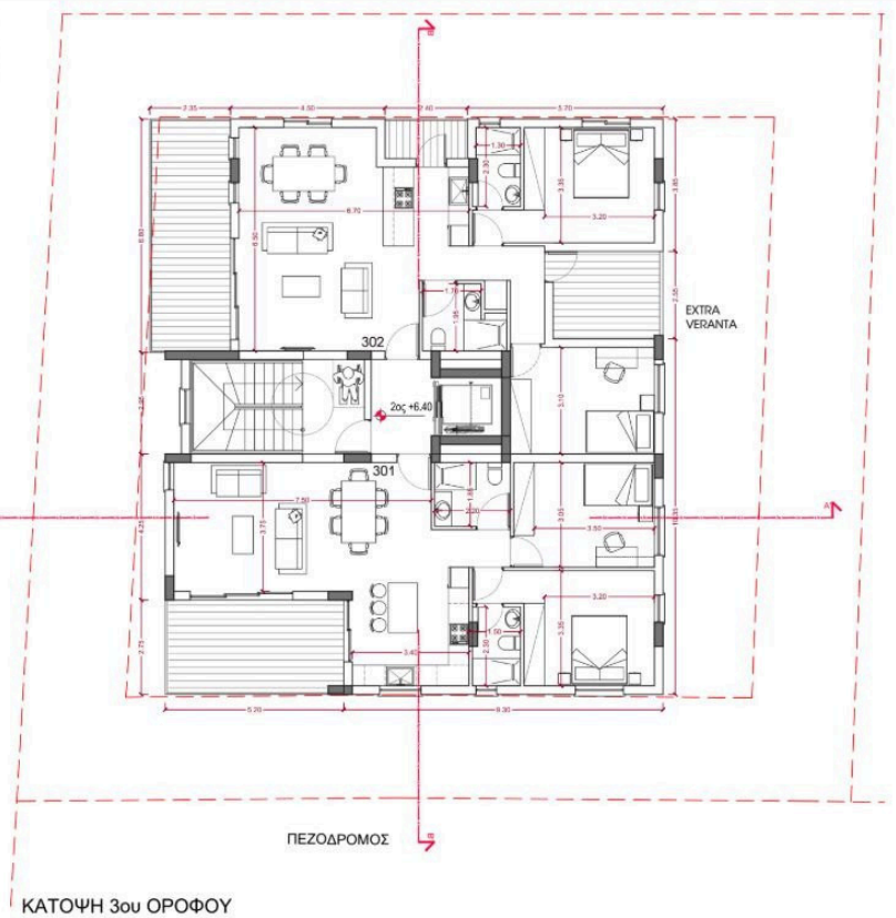
ΚΑΤΟΨΗ 3ου ΟΡΟΦΟΥ
