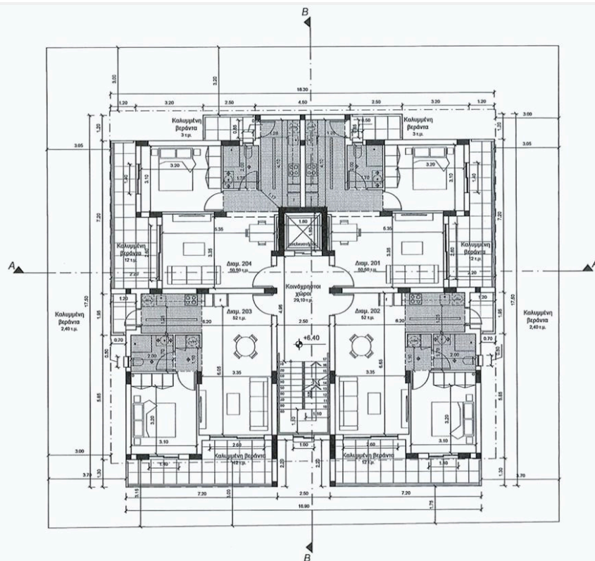
ΚΑΤΟΨΗ 2ου ΟΡΟΦΟΥ ΚΛΙΜΑΚΑ 1:100
