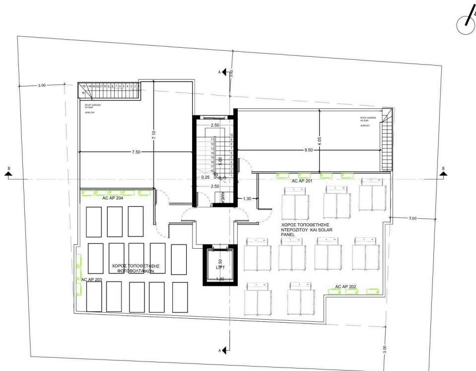
ΚΑΤΟΨΗ ΟΡΟΦΗΣ
