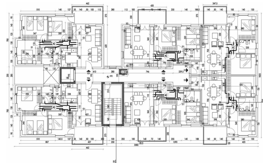
Κάτοψη ορόφου 1 1:100
