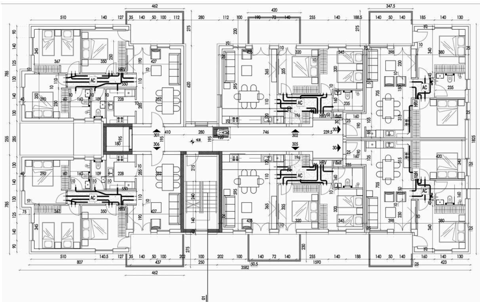
Κατοψη ορόφου 3 1 : 100
