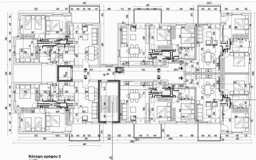
Κατοψη ορόφου 2 1 : 100
