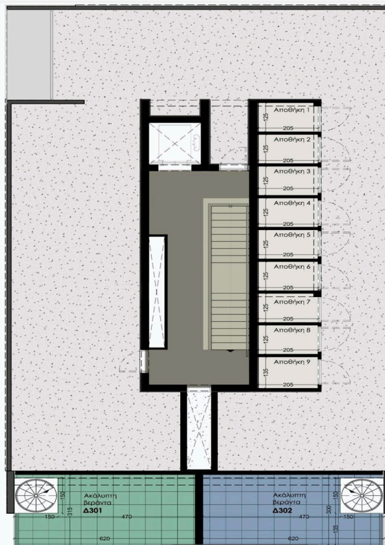
Κάτοψη Οροφής
