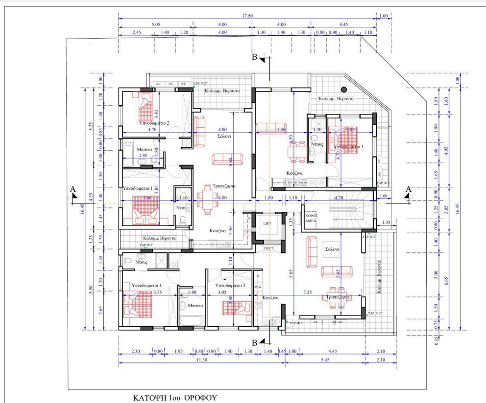
ΚΑΤΟΨΗ 1ου ΟΡΟΦΟΥ
