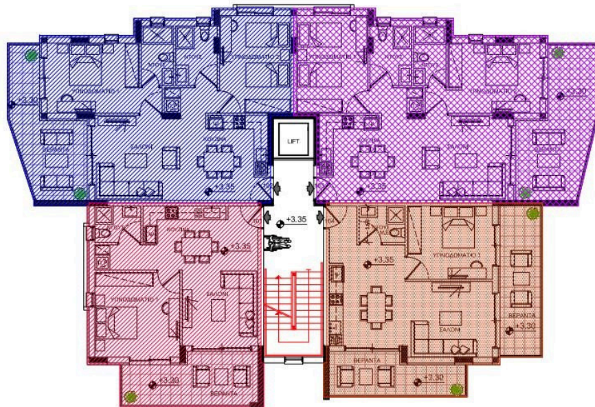
ΚΑΤΟΨΗ 1ου ΟΡΟΦΟΥ - ΔΙΑΧΩΡΙΣΜΟΣ ΚΛΙΜΑΚΑ 1:100
