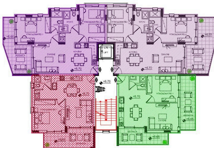
ΚΑΤΟΨΗ 2ου ΟΡΟΦΟΥ - ΔΙΑΧΩΡΙΣΜΟΣ ΚΛΙΜΑΚΑ 1:100
