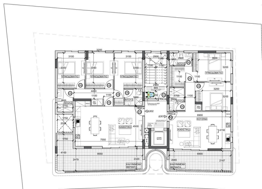
ΚΑΤΟΨΗ 3ΟΥ ΟΡΟΦΟΥ
