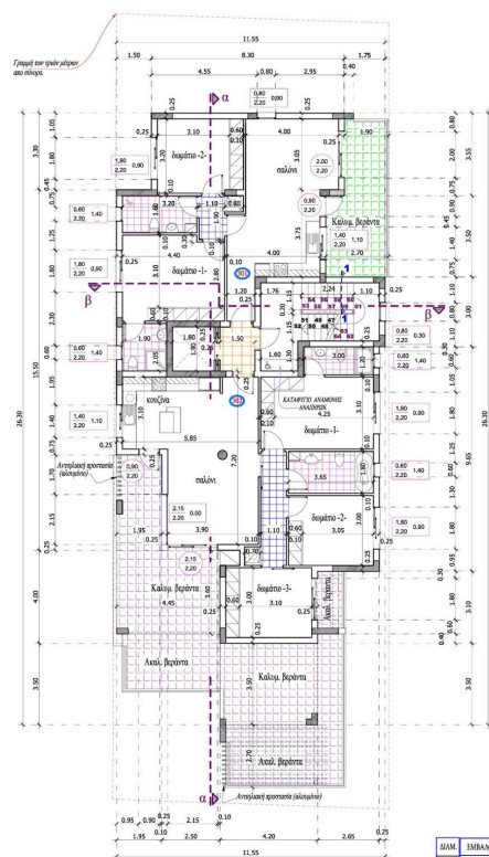
Κάτοψη 3ου ορόφου.
