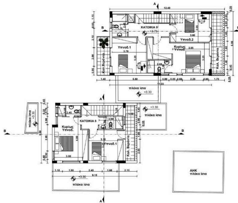
ΚΑΤΩΦΗ ΟΡΟΦΟΥ ΚΑΤΟΙΚΙΩΝ 5&6
