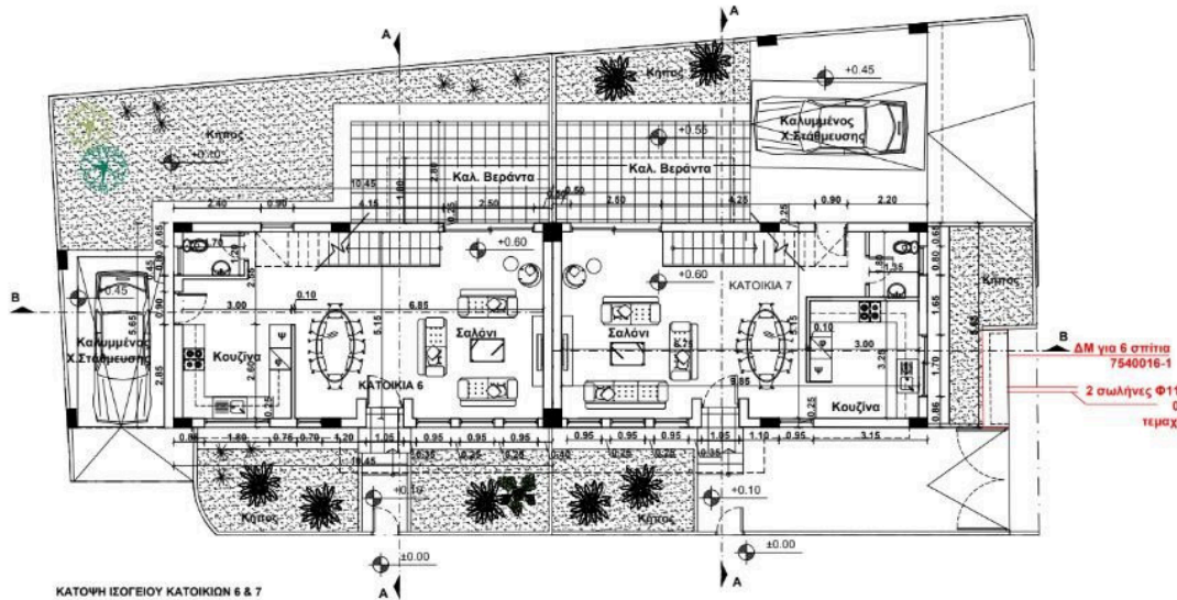
ΚΑΤΩΦΗ ΙΣΟΓΕΙΟΥ ΚΑΤΟΙΚΙΩΝ 6 & 7
