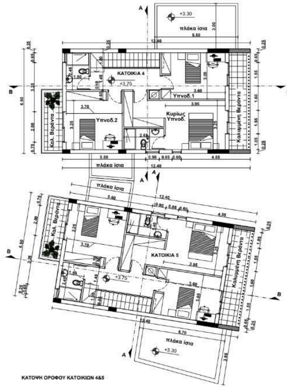
ΚΑΤΩΦΗ ΟΡΟΦΟΥ ΚΑΤΟΙΚΙΩΝ 4&5
