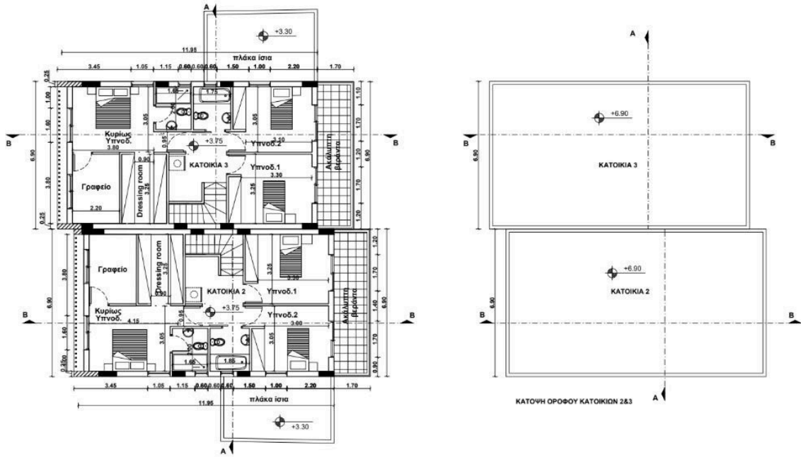
ΚΑΤΩΗ ΟΡΟΦΟΥ ΚΑΤΟΙΚΙΩΝ 263
