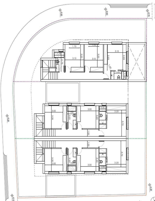
Κατόψεις ορόφου
