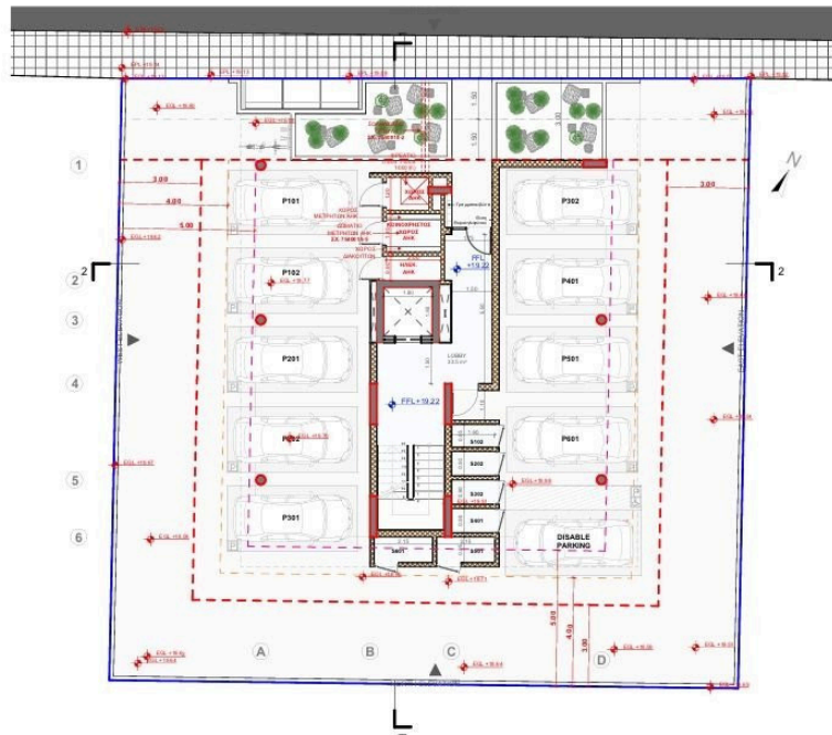
ΧΩΡΟΤΑΞΙΚΟ - ΙΣΟΓΕΙΟ ΚΛΙΜΑΚΑ 1:200
