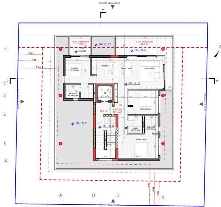
ΤΕΤΑΡΤΟΣ ΟΡΟΦΟΣ 1:200
