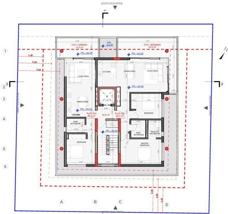
ΔΕΥΤΕΡΟΣ ΟΡΟΦΟΣ ΚΛΙΜΑΚΑ 1:200
