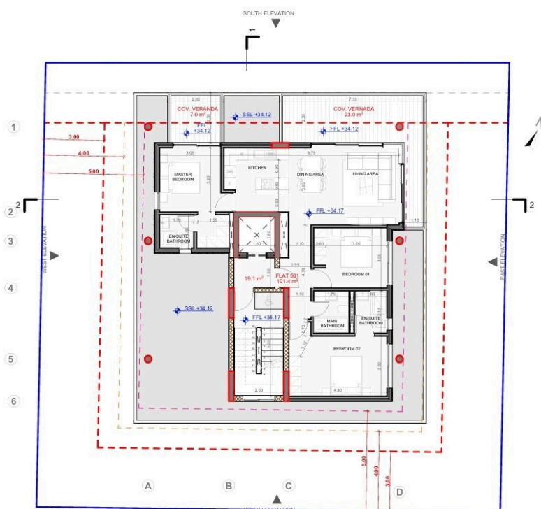
ΠΕΜΠΤΟΣ ΟΡΟΦΟΣ ΚΛΙΜΑΚΑ 1:200
