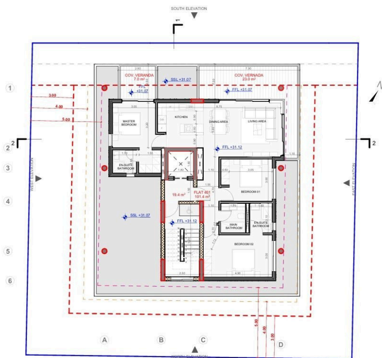
ΤΕΤΑΡΤΟΣ ΟΡΟΦΟΣ 1:200
