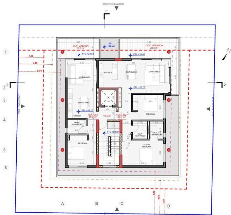
ΤΡΙΤΟΣ ΟΡΟΦΟΣ ΚΛΙΜΑΚΑ 1:200
